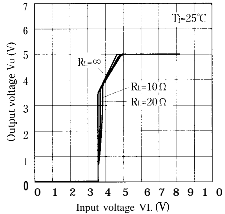
Fig. 9 Output Voltage vs. Input Voltage (PQo5sz5/PQo5sz51)
