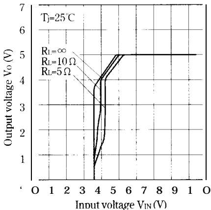
Fig. 8 Output Voltage vs. Input Voltage (PQ05SZI/PQ05SZ11)
